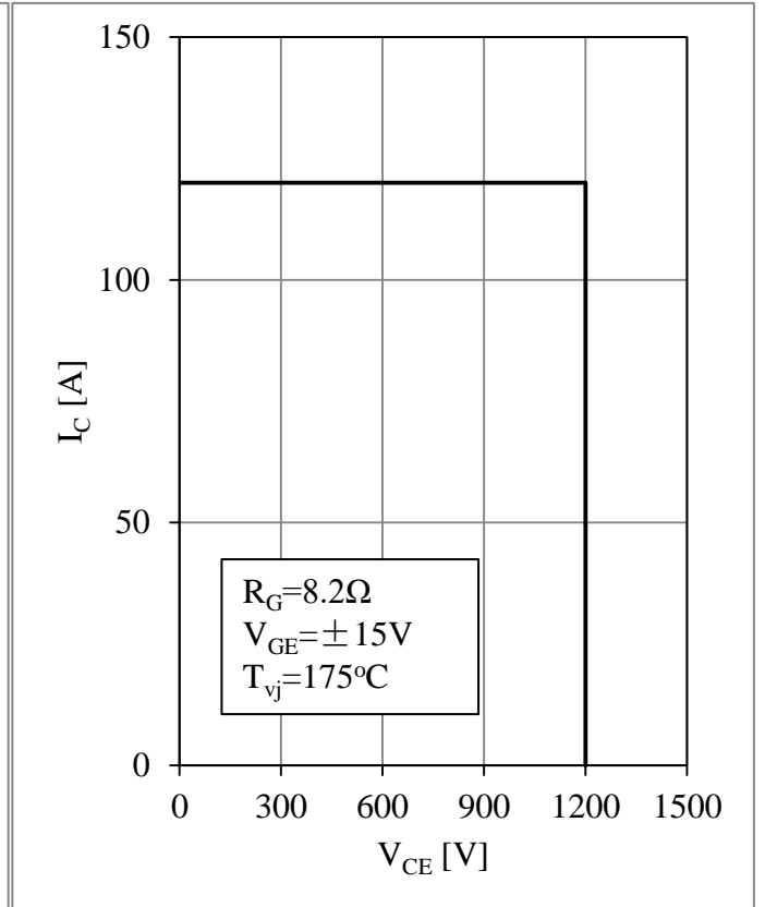
Fig 14. RBSOA
